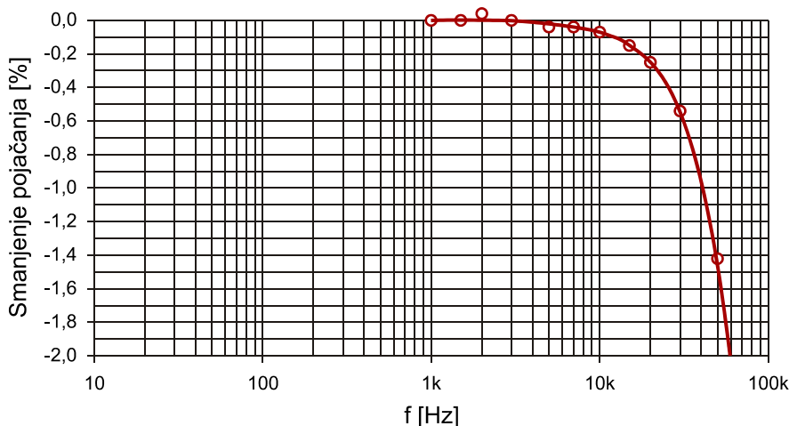
Tipičan izmereni frekventni odziv kanala pojačavača.
