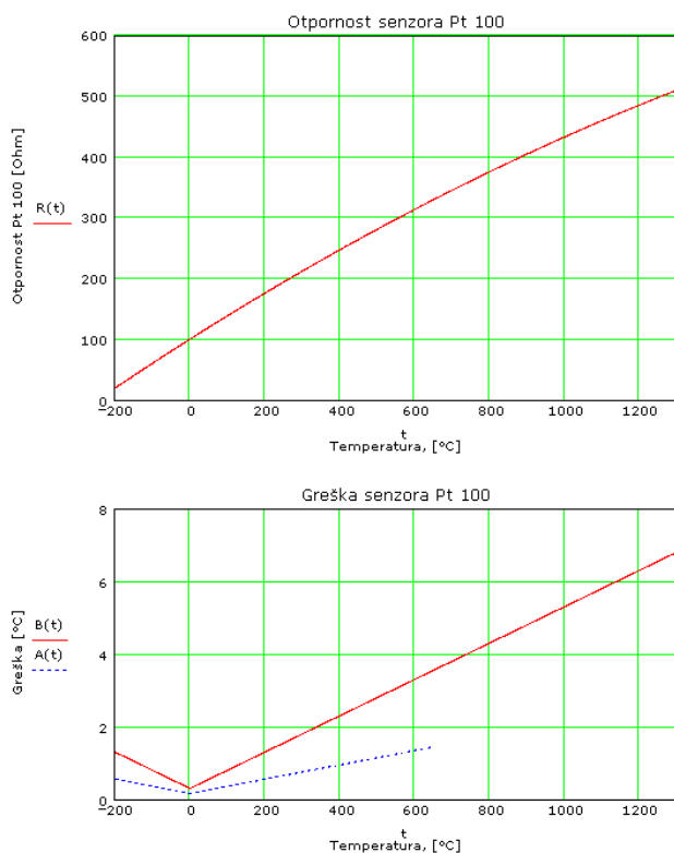
Slika 2. Za senzor Pt 100: zavisnost otpornosti od temperature i zavisnost maksimalnog modula greške od temperature.
