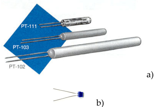
Slika 1. Senzori Pt 100: a) u staklenoj i keramičkoj enkapsulaciji (LakeShore, USA) i b) tankoslojni senzor.
